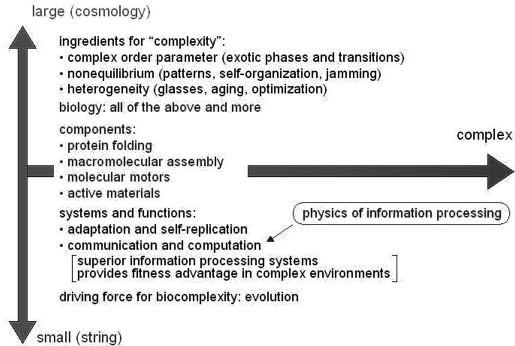
Figura 5. Diagrama sobre las Fronteras de la Física teniendo en cuenta las escalas. Entre las escalas de lo muy grande y lo muy pequeño, se sitúa el mundo de la complejidad.
